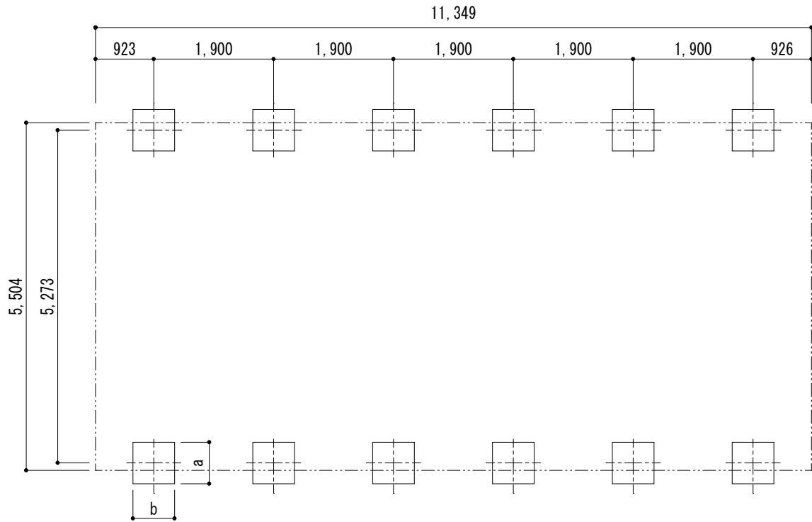
■基礎配置図
